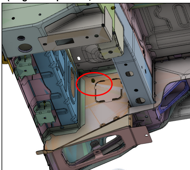
Perno 22 (furgão Propulsion, chassis-cabina e cabina dupla)
