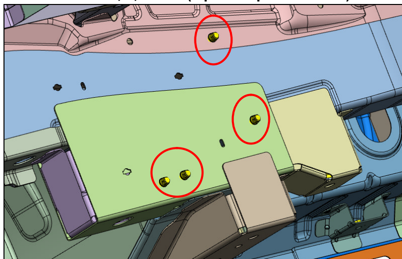
Pernos 7, 8, 9 e 10 (4 pernos para E-TECH):
