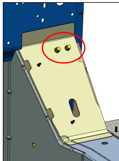
Perno 22 (furgão Propulsion, chassis-cabina e cabina dupla)
