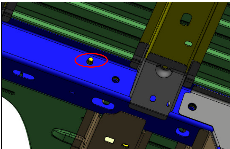
Perno 30 (qualquer tipo, exceto furgão Propulsion)
