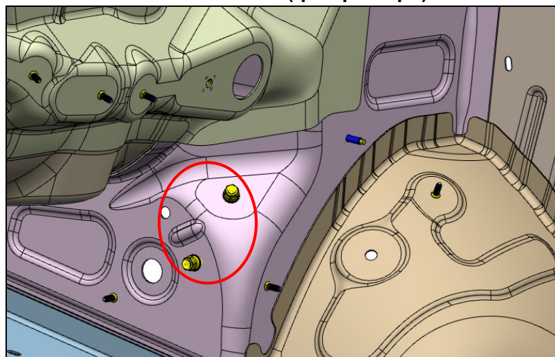
Pernos 28 e 29 (qualquer tipo)
