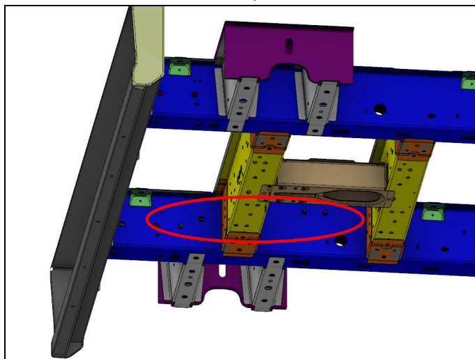
Pernos 34, 35 e 36
